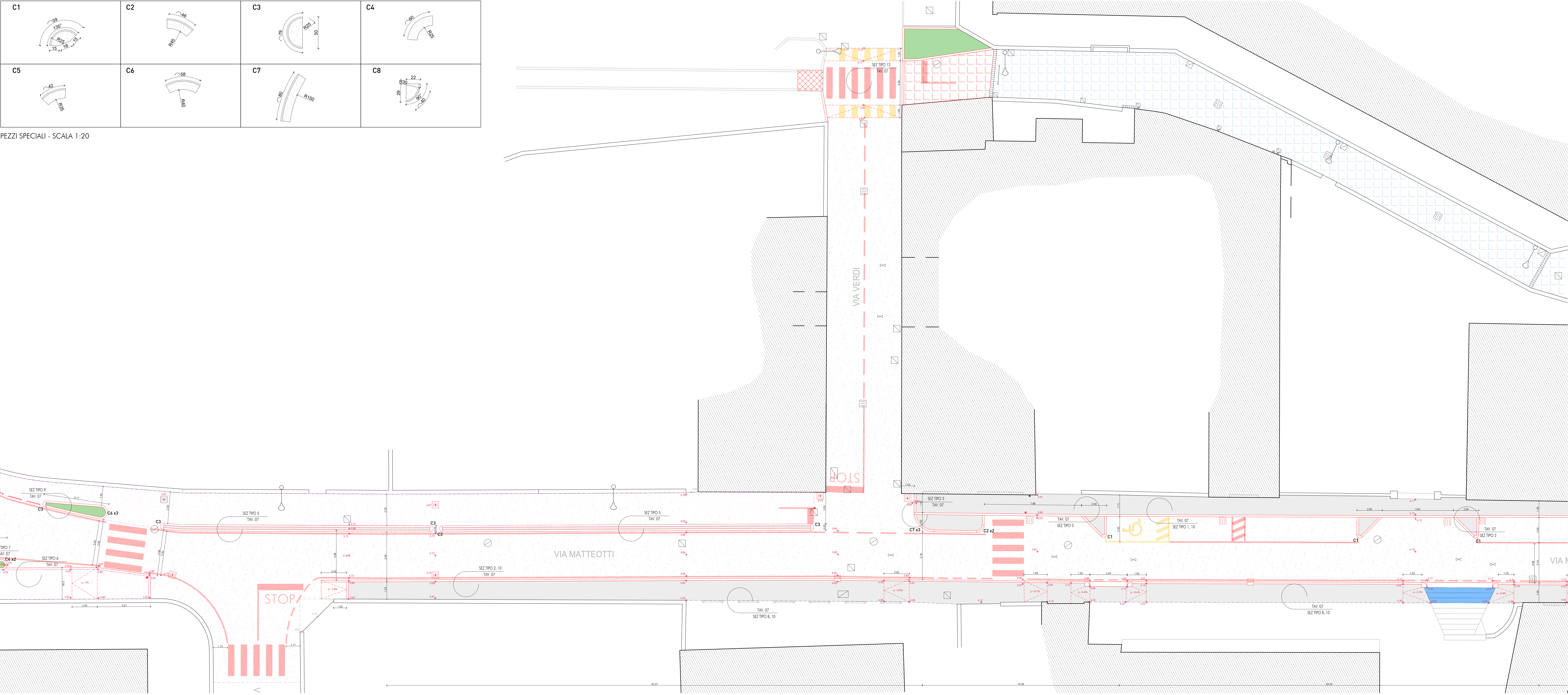
PLANIMETRIA - SCALA 1:100
